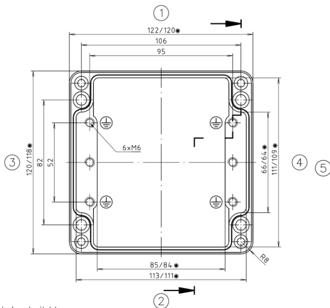
Unterteil / base
