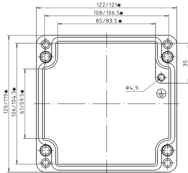
Deckel / lid
