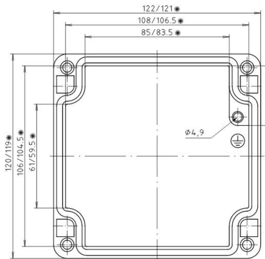
Deckel / lid
