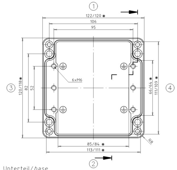
Unterteil / base
