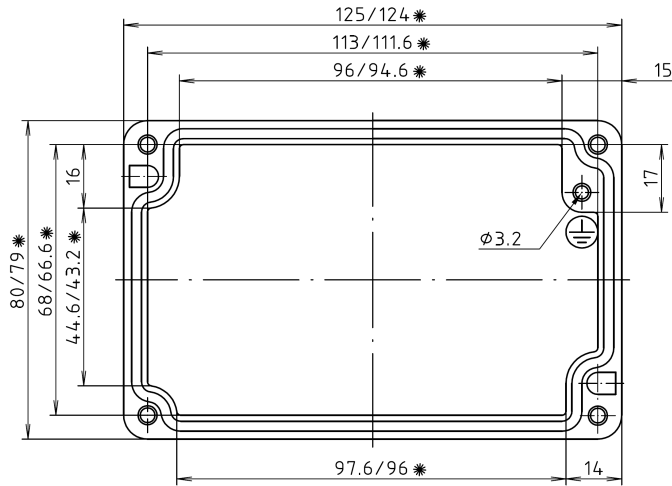
Deckel / lid
