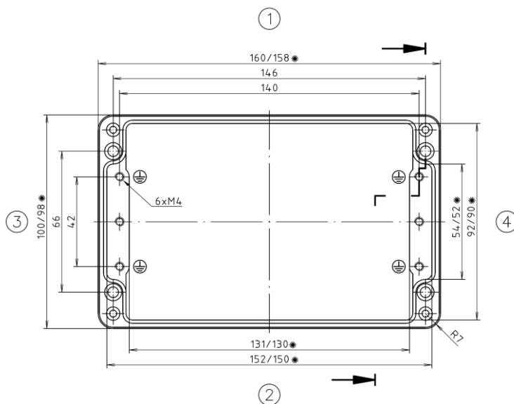
Unterteil / base
