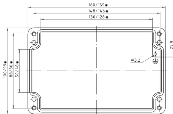
Deckel / lid
