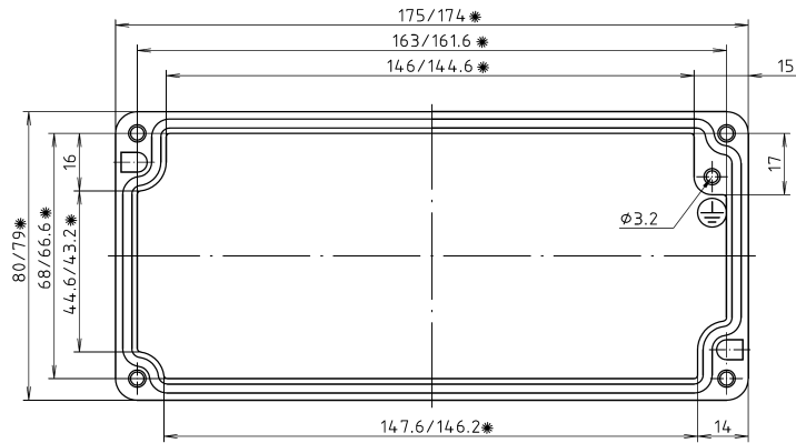
Deckel / lid
