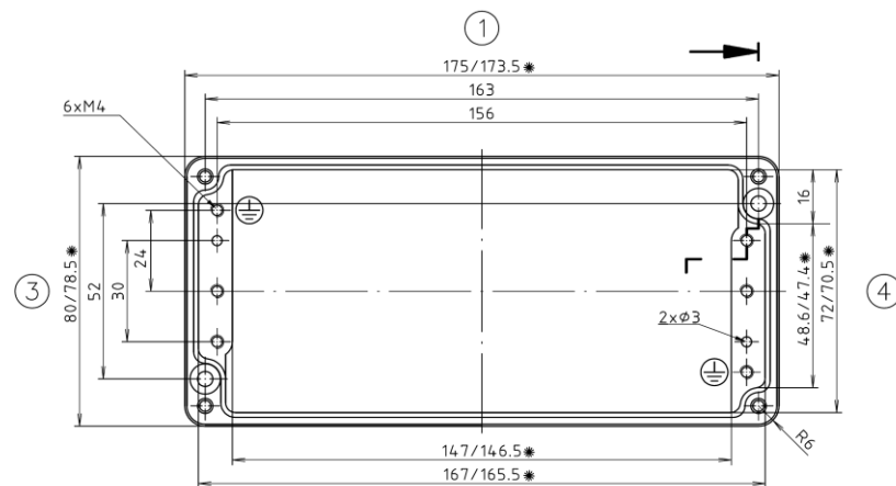
Unterteil / base
