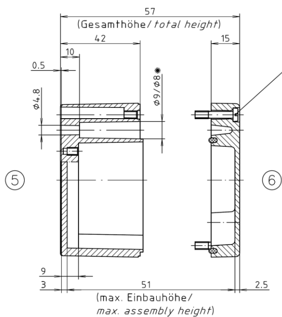
Unterteil / base
