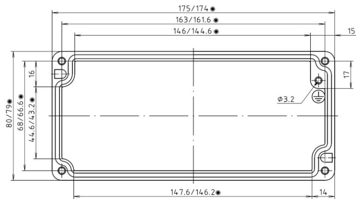
Deckel / lid
