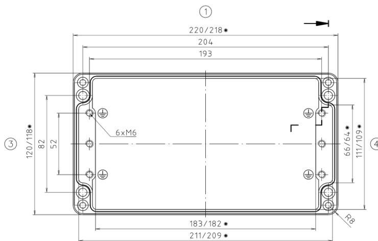
Unterteil/ base
