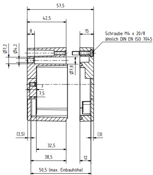
A-A ( 1 : 1 )
