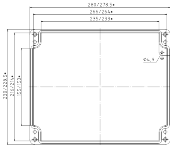
Deckel/ lid
