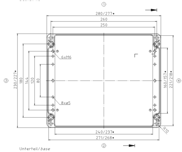
Unterteil/ base
