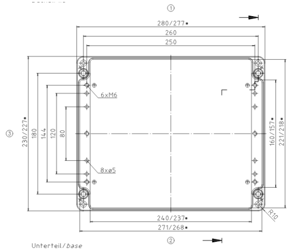
Unterteil/base
