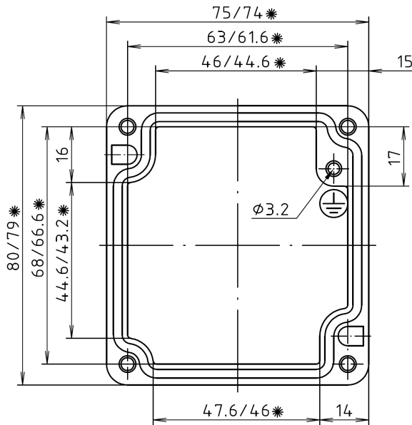
Deckel / lid
